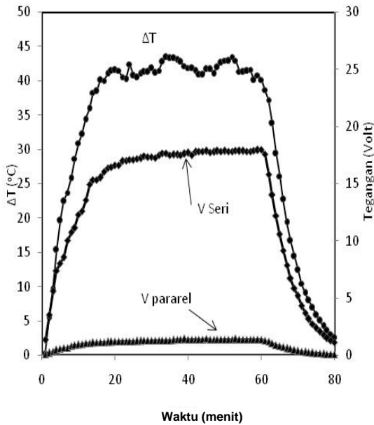
Gambar 6. Grafik Karakter Termoelektrik dengan Tegangan Input Pemanas 220V
