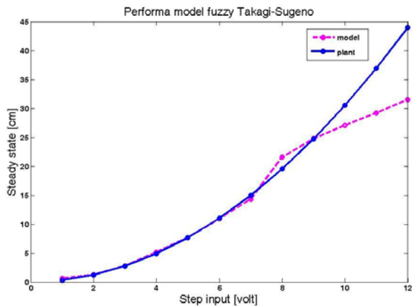
Gambar 6. Kinerja model terhadap masukan fungsi step
