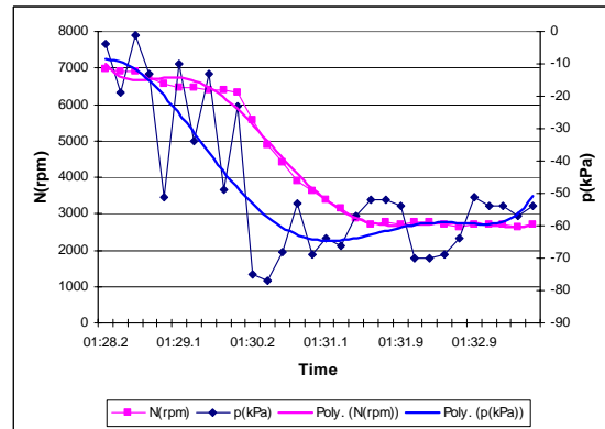
Gambar 12. Karakteristik Intake Manifold saat Deselerasi
