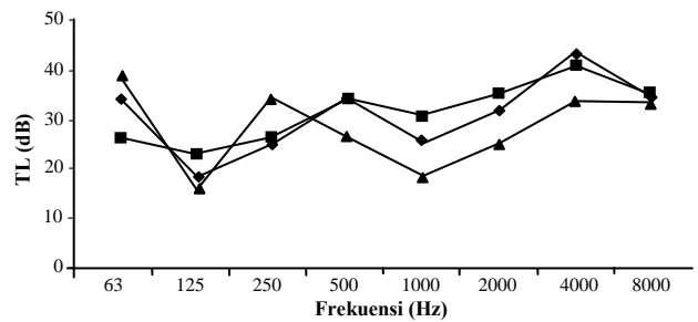
Gambar 3. Nilai STL 2 (Dua) Lapis Bahan Uji Untuk Tiap Frekuensi, Plywood+Tray (♦), Plywood+Busa (■), Plywood+Busa+Sabut (▲)
