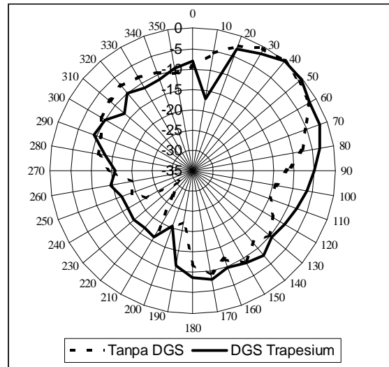
Gambar 10. Hasil pengukuran pola radiasi medan E antenna
