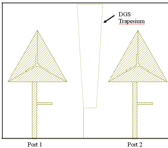
Gambar 5. Konfigurasi antenna untuk memperoleh nilai mutual coupling
