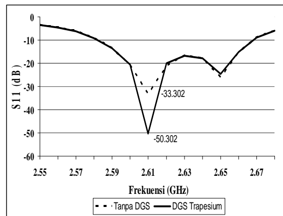
Gambar 3. Hasil simulasi return loss
