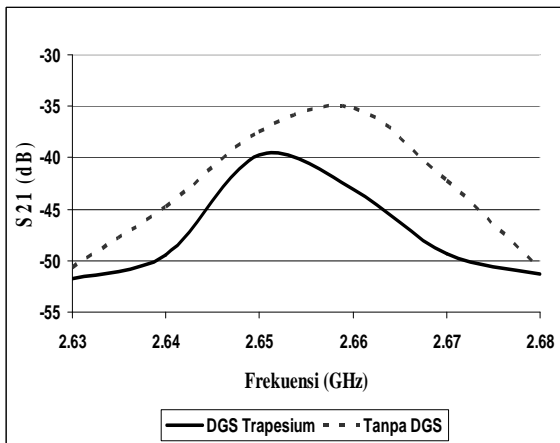
Gambar 9. Hasil pengukuran mutual coupling
