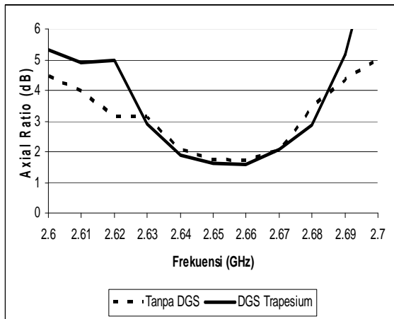
Gambar 8. Hasil pengukuran axial ratio
