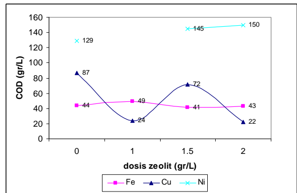
Gambar 9. Pengaruh konsentrasi zeolit terhadap kadar COD akhir
