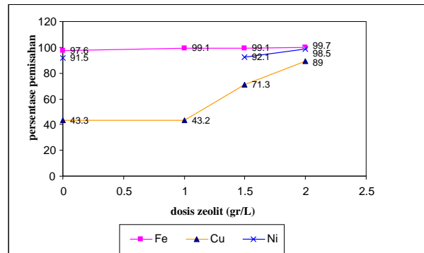
Gambar 8. Pengaruh konsentrasi zeolit terhadap persentase pemisahan logam
