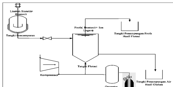
Gambar 2. Skema alat untuk flotasi dengan diffuser udara-ozon dari oksigen
