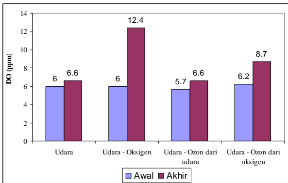
Gambar 7. Perbandingan Nilai DO Larutan Akhir Flotasi Antar Diffuser
