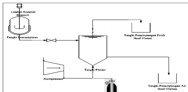
Gambar 3. Skema alat untuk flotasi dengan diffuser udara-oksigen
