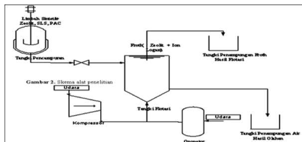
Gambar 1. Skema alat untuk flotasi dengan diffuser udara-ozon dari udara
