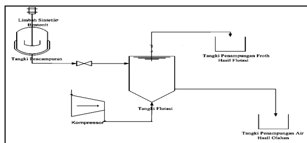
Gambar 4. Skema alat untuk flotasi dengan diffuser udara
