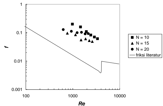
Gambar 7. Variasi faktor friksi, f , terhadap bilangan Reynolds, Re .
