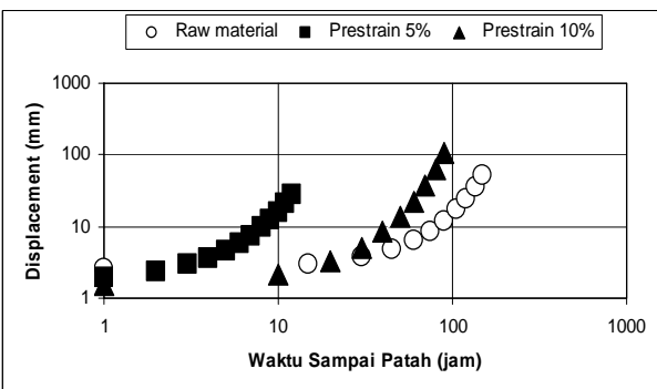
Gambar 3. Hubungan displacement terhadap waktu sampai patah dengan \sigma_{statis} = 369,6 Mpa.
