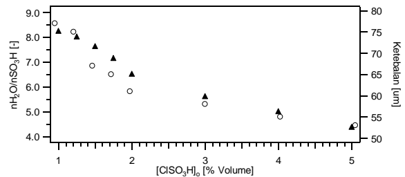
Gambar 4. Pengaruh konsentrasi \text{ClSO}_3\text{H} terhadap (○) jumlah molekul air per gugus asam sulfonat dan (▲) ketebalan membran. Sulfonasi dilakukan pada suhu kamar selama 8 jam.
