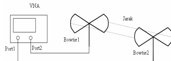
Gambar 5. Skema pengukuran S_{21} dengan VNA
